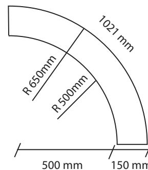
CURVA GRANDE
