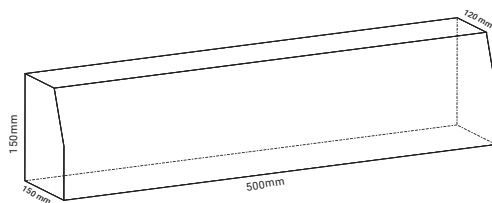
MODULO RIBASSATO
