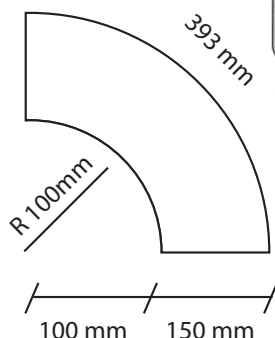
CURVA PICCOLA
